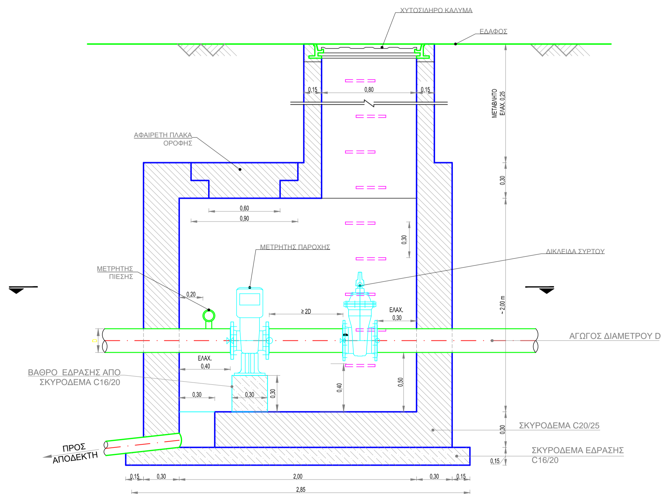
ΤΟΜΗ Α-Α
