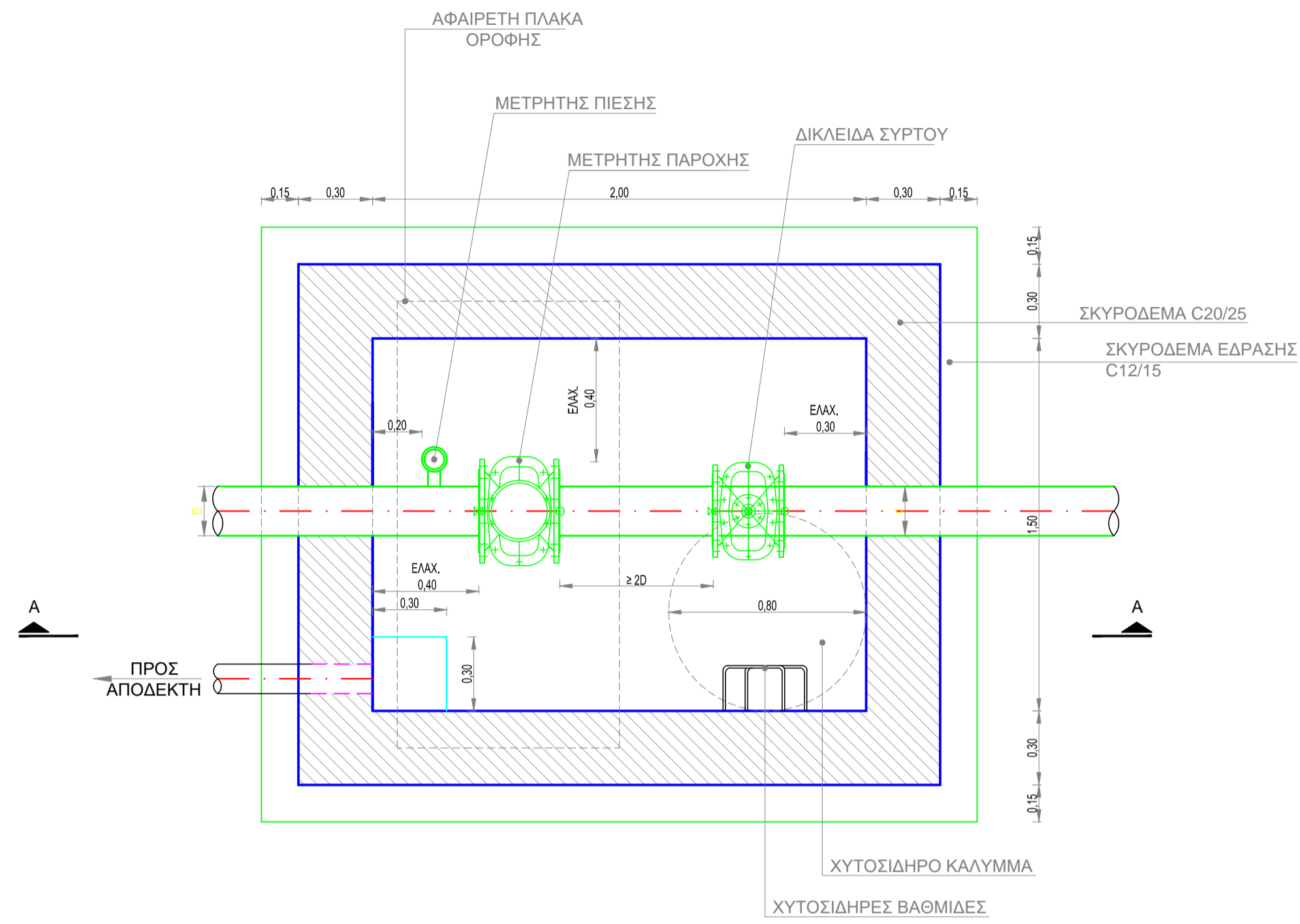
ΚΑΤΟΨΗ
