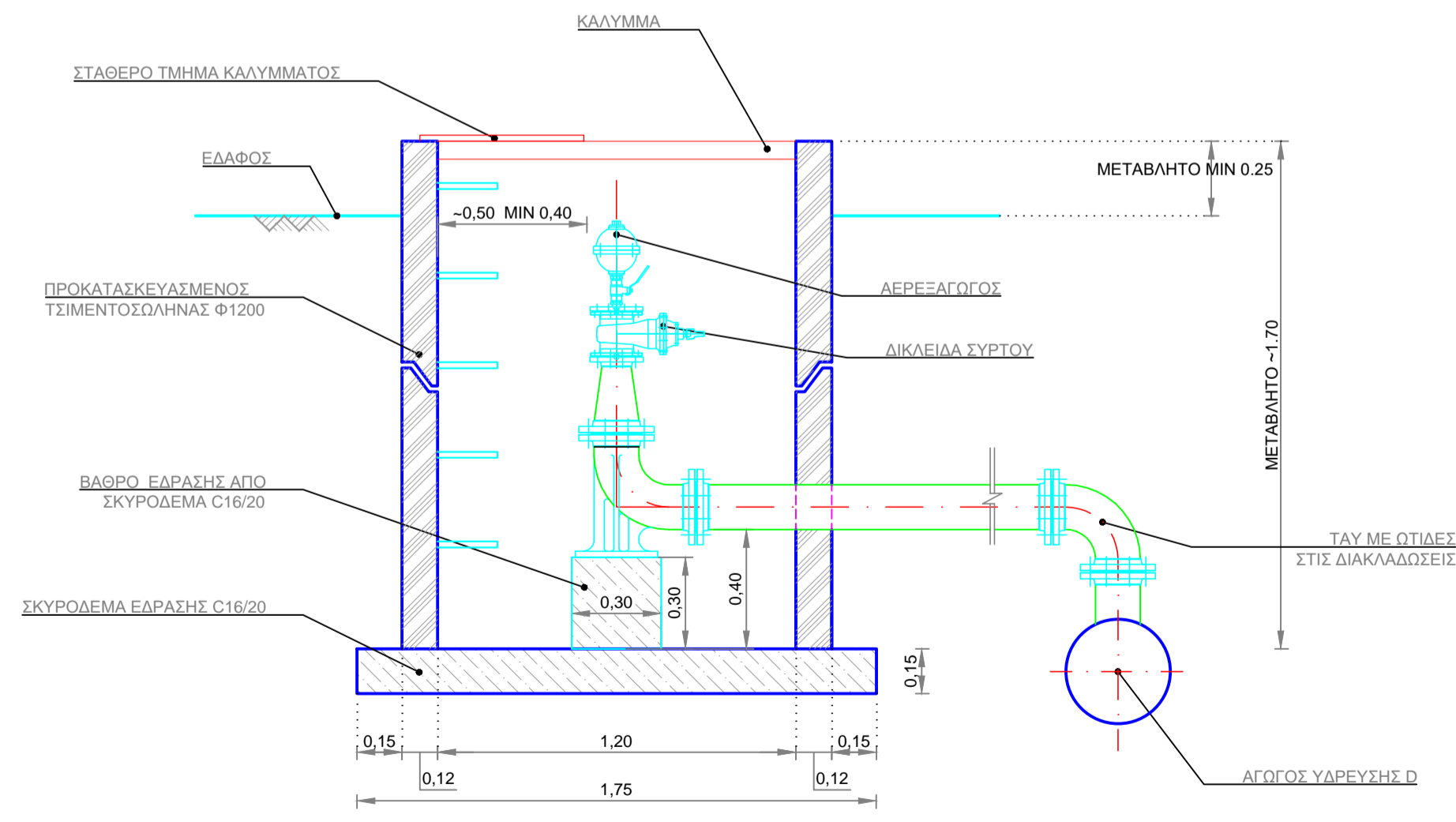
ΤΟΜΗ Α-Α
