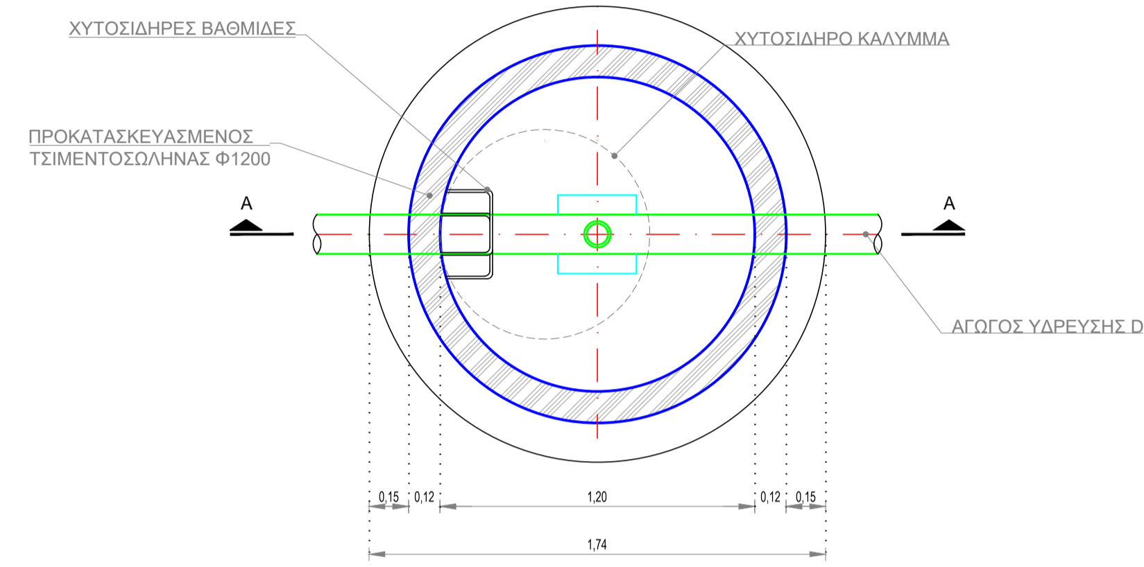
ΚΑΤΟΨΗ
