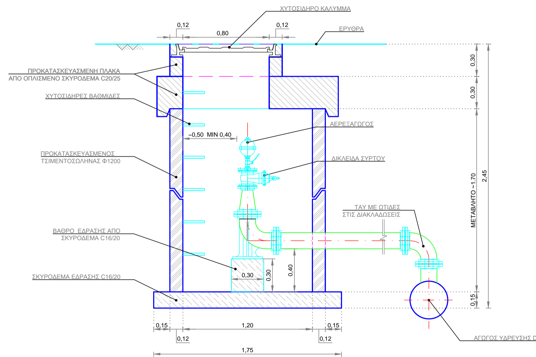
ΤΟΜΗ Α-Α
