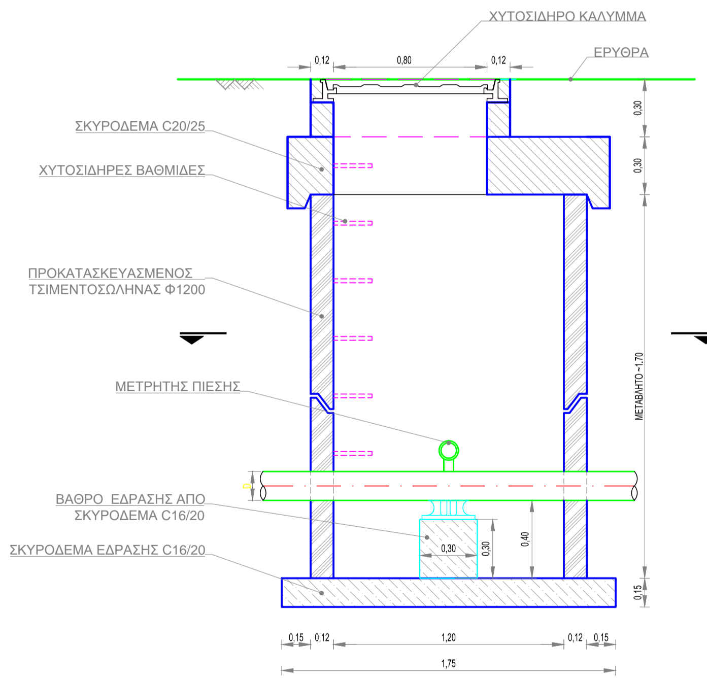
ΤΟΜΗ Α-Α
