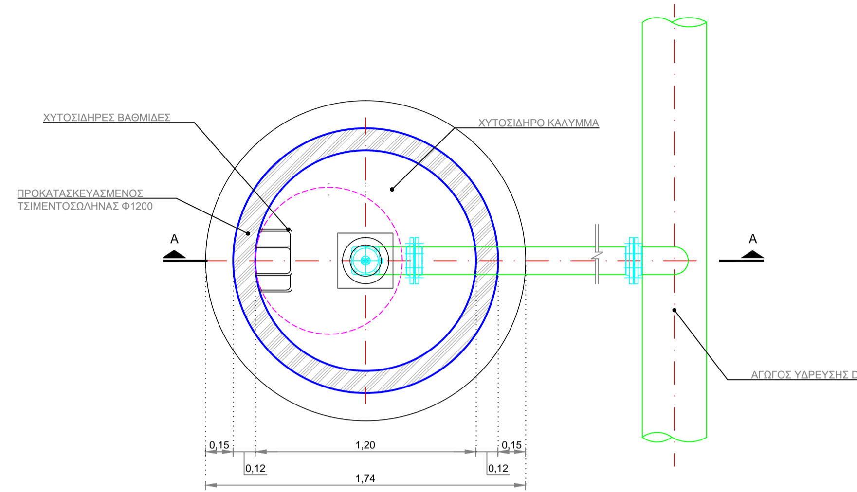
ΚΑΤΟΨΗ
