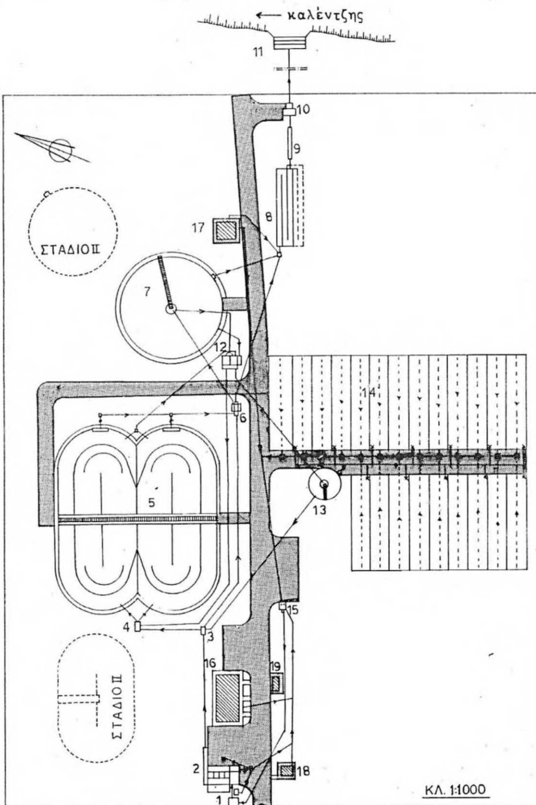
Σχήμα: Κάτοψη ΕΕΛ Καρδίτσας
